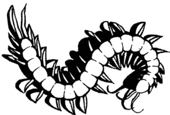
centipede
